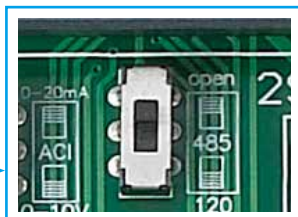
RS-485 通訊
